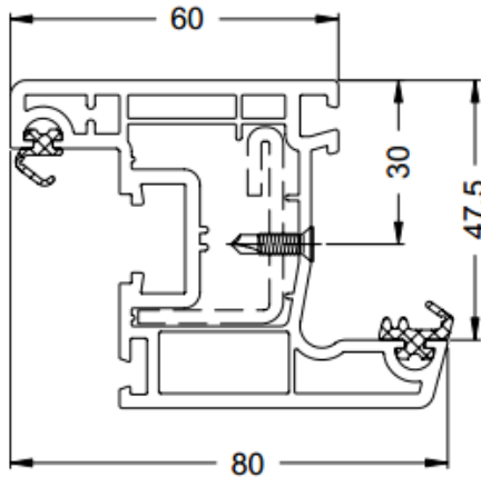
Крепление усиленного профиля
