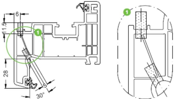
Водоотвод и вентиляция створки Classic
