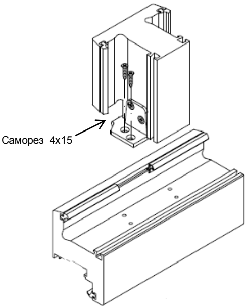
Установка импоста в створку
