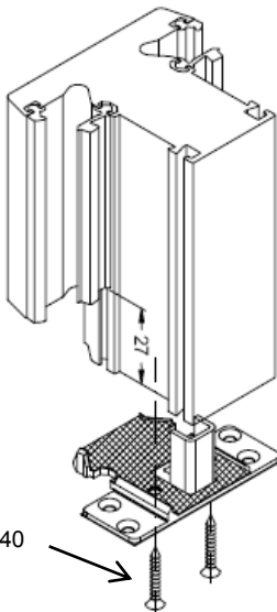
Фальцевый соединитель
