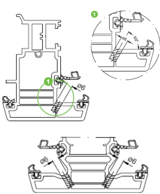
Вентиляция
