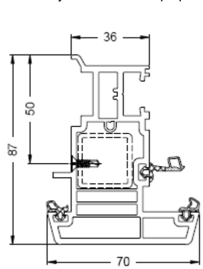
Крепление усилительного профиля
