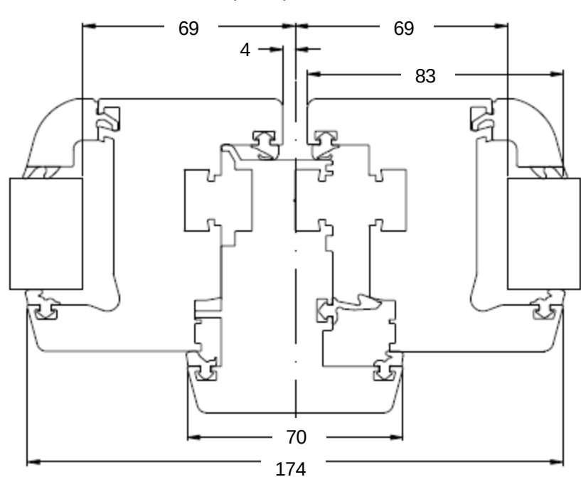
Размер до фальца стекла
