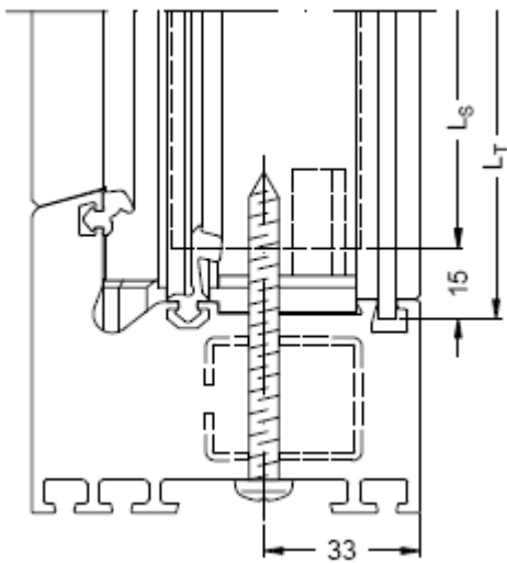
Раскрой стали = размер импоста – 30 мм Ls = Lt - 30
