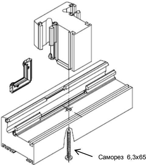
Установка импоста с рамным соединителем
