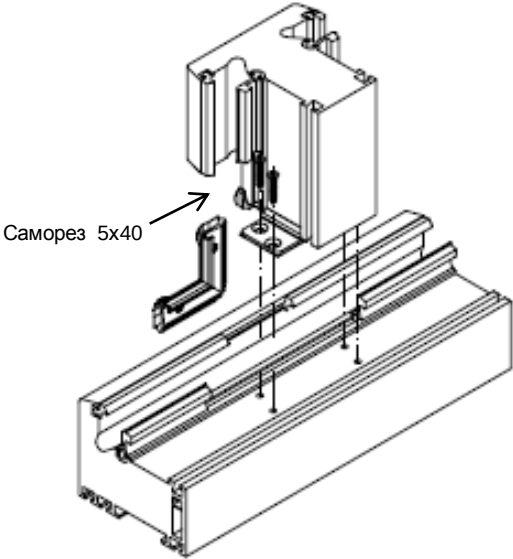
Установка импоста с фальцевым соединителем
