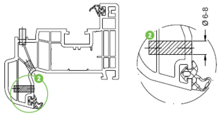
Водоотвод и вентиляция створки Rondo
