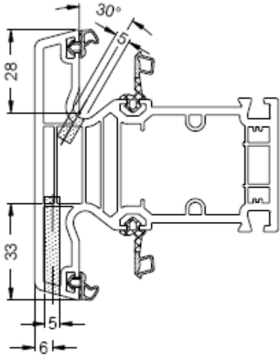
Водоотвод и вентиляция
