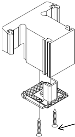
Рамный соединитель
