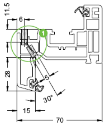
Водоотвод и вентиляция створки Classic
