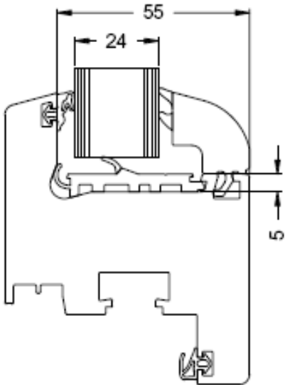
Вкладыш фальца для вклеивания стеклопакета
