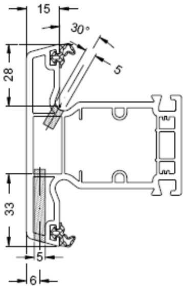
Водоотвод и вентиляция
