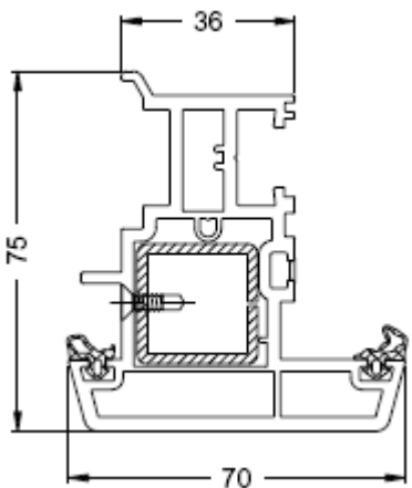
Крепление усиленного профиля
