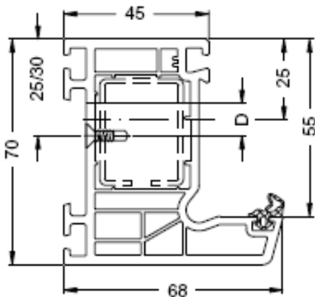
Крепление усилительного профиля
