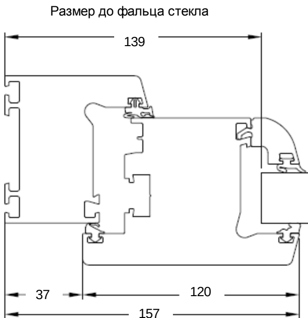
Водоотвод и вентиляция створки Rondo
